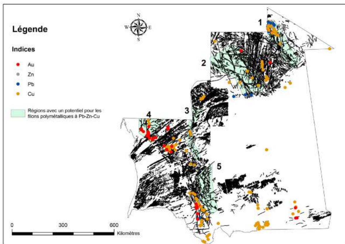
Figure 15: Zones favorables pour des dépôts de veines polymétalliques Pb-Zn-Cu en surimposition sur le fond de carte structurale au 1/500 000
