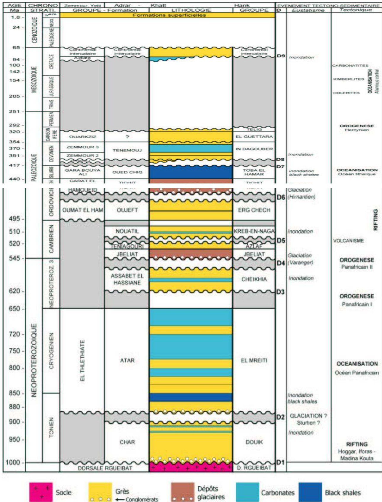
Figure 8. Colonne stratigraphique synthétique des formations Protérozoïques et Paléozoïques de la partie Nord du Bassin de Taoudéni.
