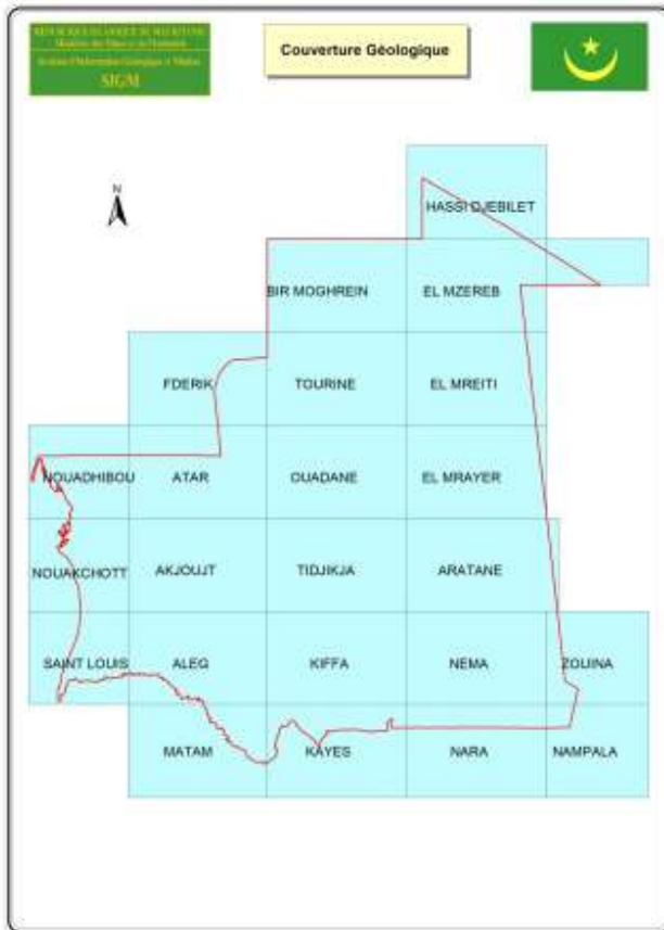
Figure 2 : Couverture géologique: Couverture totale de la Mauritanie au 1/500.000ème
