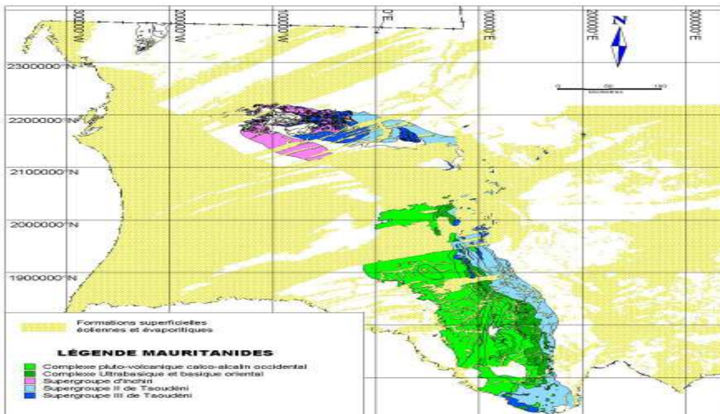
Figure 9. Carte géologique de la Chaîne des Mauritanides.
